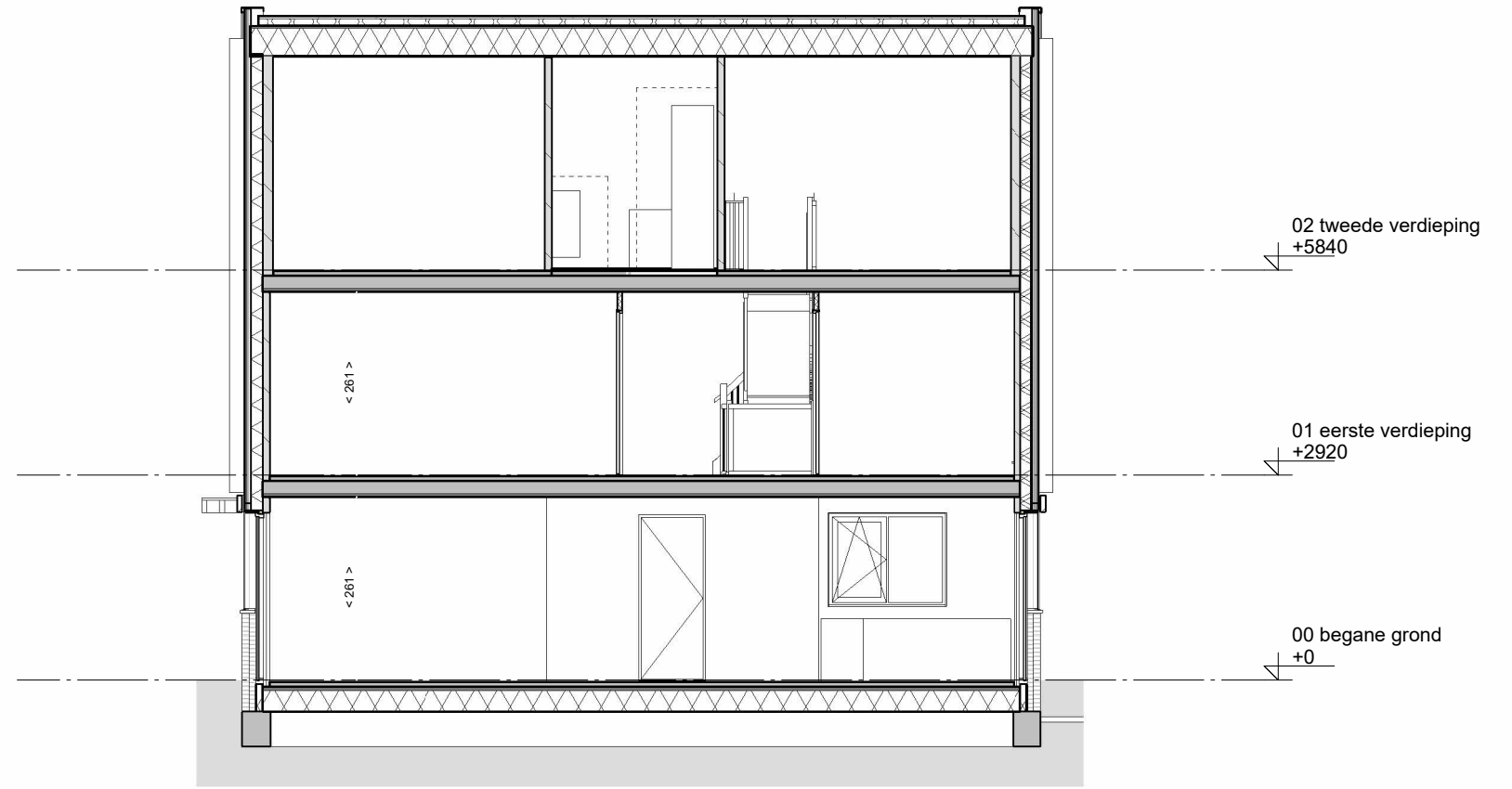
dwarsdoorsnede
