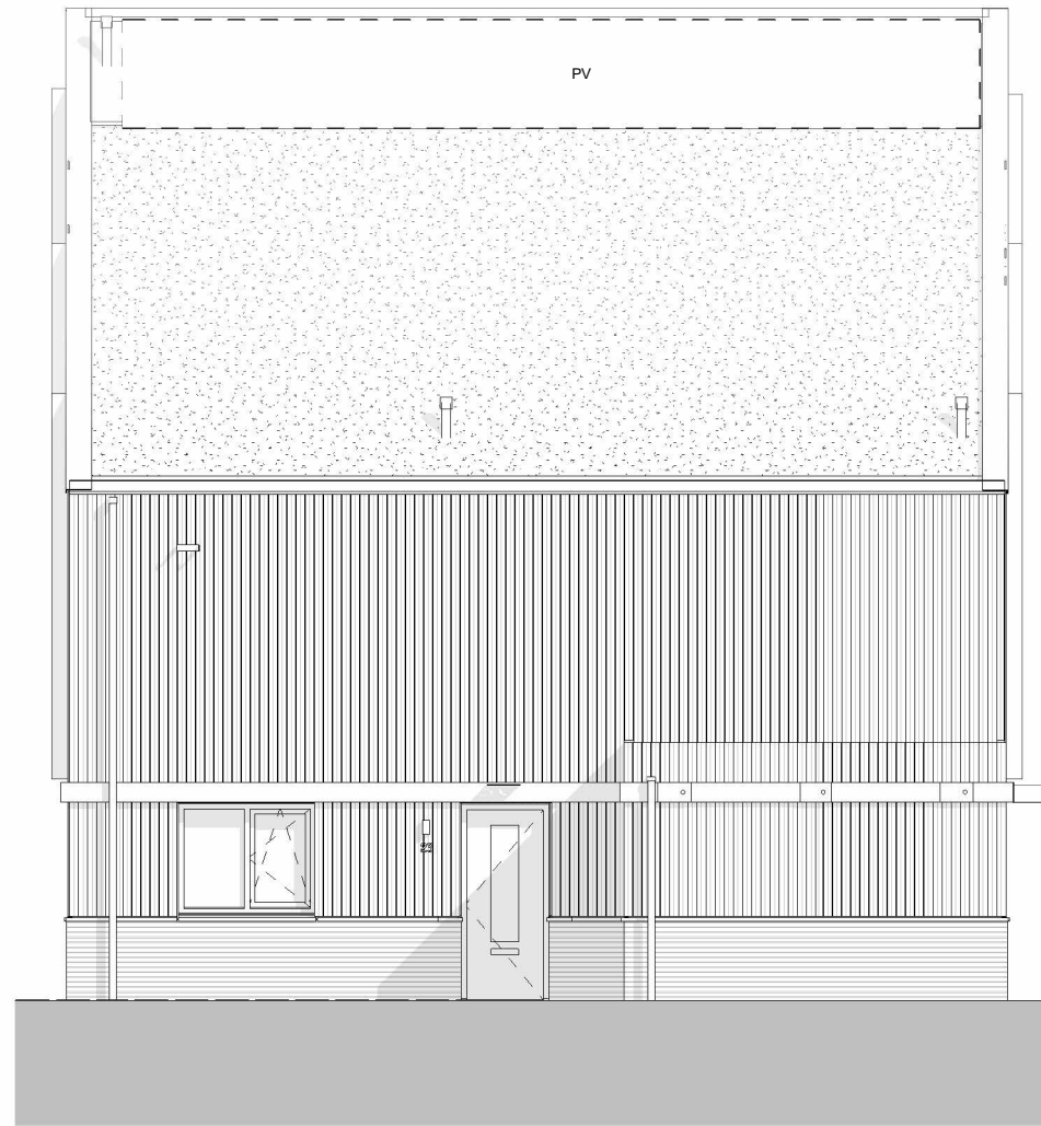
zijgevel (noordoost)
